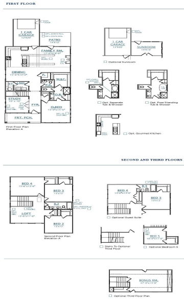
ELEVATION A
